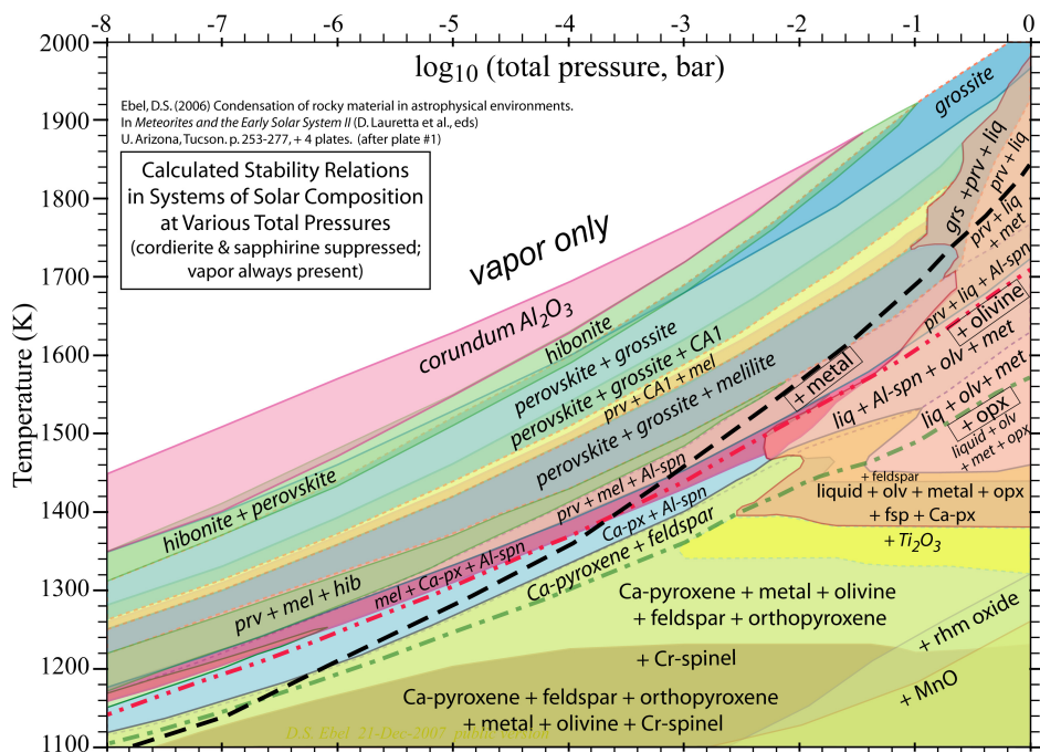
Obr. 69 — Fázový diagram T(P) (tj. transponovaný P(T) ) pro pevnou látku deponovanou, kondenzovanou či utuhlou při různých tlacích. Počáteční složení opět odpovídá fotosféře. Kromě minerálů, resp. jejich skupin, zmiňovaných výše, jsou zde uvedeny: skupina melilitu, tj. gehlenit \text{Ca}_2\text{Al}_2\text{SiO}_7 , ākermanit \text{Ca}_2\text{MgSi}_2\text{O}_7 ; spinely, spinel \text{MgAl}_2\text{O}_4 , chromit \text{FeCr}_2\text{O}_4 ; olivíny, forsterit \text{Mg}_2\text{SiO}_4 , fayalit \text{Fe}_2\text{SiO}_4 ; pyroxeny, enstatit \text{Mg}_2\text{Si}_2\text{O}_6 , ferosilit \text{Fe}_2\text{Si}_2\text{O}_6 ; wollastonit \text{Ca}_2\text{Si}_2\text{O}_6 ; živce, anortit \text{CaAl}_2\text{Si}_2\text{O}_8 , albit \text{NaAlSi}_3\text{O}_8 , ortoklas \text{KAlSi}_3\text{O}_8 . Převzato z http://research.amnh.org/~debel/vapors1/vapors1.html .
