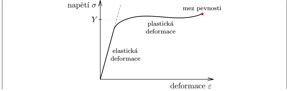
Obr. 11 — Typická závislost mezi napětím \sigma a deformací \varepsilon pro pevné látky. První oblast, elastičká, je přibližně lineární, \sigma = E\varepsilon . Druhá oblast je plastická, ve které \varepsilon roste i při stálém (velkém) \sigma \simeq Y .
