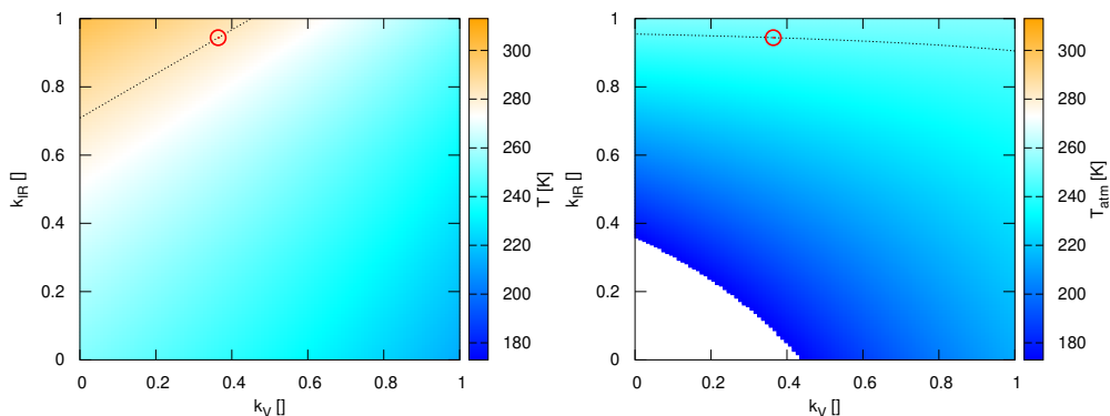
Obr. 41 — Teplota Země T (vlevo) a atmosféry T_{atm} (vpravo) v závislosti na absorpčním koeficientu k_V ve viditelné a k_{IR} v infračervené oblasti spektra. Červený bod odpovídá našemu měření.
