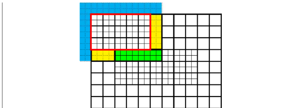
Obr. 7 — Duchářská oblast v okolí zjemnělé sítě, která se vyplňuje z okrajové podmínky (modře), z jednoho sousedního bloku se stejným rozlišením (žlutě) a z dvou sousedních bloků s odlišným rozlišením (zeleně). Převzato z [6].
