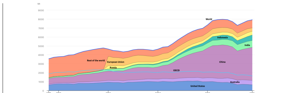
Obr. 44 — Roční těžba uhlí v megatunách (Mt) v období let 1978 až 2019 podle IEA. Převzato z https://www.iea.org/ .
