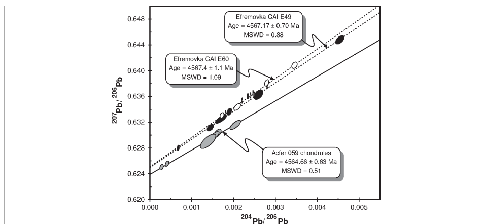
Obr. 64 — Isochróna Pb/Pb pro vápenato–hlinité inkluze (CAI) z meteoritu Efremovka, vykazující stáří (4,567 \pm 0,001) Gyr. Pro porovnání jsou zobrazeny chondrule z meteoritu Acfer 059, se stářím asi o 0,003 Gyr menším. Převzato z [82].
