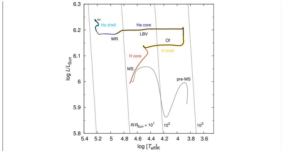
Obř. 101 — HR diagram pro hvězdu s počáteční hmotností M = 85 M_{\odot} . Metalicita byla volena Z = 0,02 , opacity dle Grevesse a Sauval (1998) pro látku obohacenou o C/O (tzv. typ 2), účinnost větru \eta = 0,8 (dle Vink aj. 2001, Nugis a Lamers 2000), parametr konvekce \alpha = 1,5 (dle Henyey aj. 1965), dále bylo použito Ledouxovo kritérium, parametr semikonvekce \alpha_{\text{semi}} = 0,01 , termohalinní cirkulace \alpha_{\text{th}} = 2 (Kippenhahn aj. 1980), přestřelování \alpha_{\text{ov}} = \alpha , s exponenciální poklesem popsáním f_0 = 0,0005 , f_{\text{ov}} = 0,001 . Na grafu je zobrazen relativně malý rozsah zářivých výkonů. Hvězda nepostoupila ani do fáze RGB mimo jiné díky ztrátě hmoty způsobené větrem.
