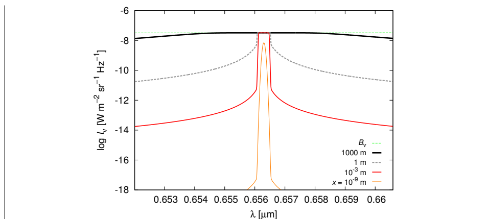
Obr. 50 — Přenos záření I_\nu(x) pro dvouhladinový atom, konkrétně přechod odpovídající čáře H_\alpha , \lambda_{12} = 656,3 \text{ nm} , E_{12} = hc/\lambda_{12} = 1,8941 \text{ eV} , Einsteinovy koeficienty A_{21} = 6,4651 \cdot 10^7 \text{ s}^{-1} , B_{21} = B_{12} = 1,0968 \cdot 10^{21} \text{ J}^{-1} \text{ m}^2 \text{ sr} . Teplota byla T = 5780 \text{ K} , hustota \rho = 10^{-9} \text{ kg m}^{-3} (tzn. asi jako fotosféra). Při LTE jsou populace hladin dány Boltzmannovým vztahem, n_2/n_1 = \exp[-E_{12}/(kT)] = 0,02238 , celková koncentrace n = n_1 + n_2 = \rho/(\mu m_H) . Použita byla aproximace Voigtova profilu \phi_{12}(\nu) , kde Gaussův profil pro termální rozšíření měl parametr \sigma = 0,02 \text{ nm} a Lorentzův profil pro srážkové rozšíření \gamma = 5 \cdot 10^{-10} \text{ nm} . Okrajová podmínka byla I_\nu(0) = 0 . Nejprve je čára emisní, postupně roste, ale maximálně do úrovně kontinua dané zdrojovou funkcí S_\nu . Jádru čáry je kompaktní, teprve křídla způsobují postupné rozšiřování profilu a přechod ke kontinuu.
