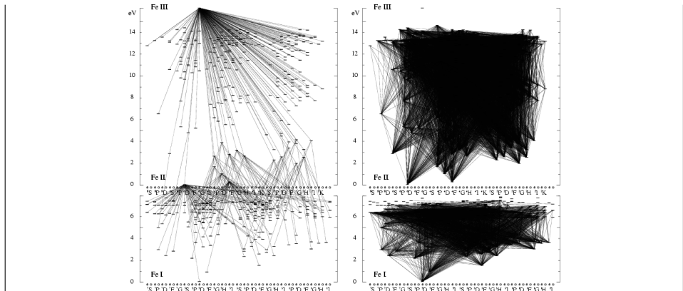
Obr. 52 — Grotrianův diagram pro železo Fe I, Fe II a Fe III. Na vodorovné ose jsou vyznačeny různé kvantové stavy atomů, na svislé jemu příslušná energie E_{ij} , každá spojnice vyznačuje možný energetický přechod. Převzato z Gehren aj. (2000).
