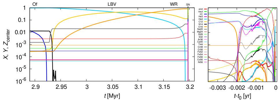
Obr. 103 — Abundance v centru (pro M = 85 M_{\odot} ) a detail těsně před explozí SN, se škálou v rocích. Po přeměně He na C/O velmi rychle proběhne série reakcí, kdy zachycováním částic \alpha vzniknou jádra se sudým Z a N = Z , tj. zejména ^{52}\text{Fe} , ^{56}\text{Ni} , který se ovšem záhy rozpadá dvakrát \beta^+ . Při vzniku jádra ^{56}\text{Fe} se vývoj odehrává na škále hodin; samotný kolaps poté na škále sekund.
